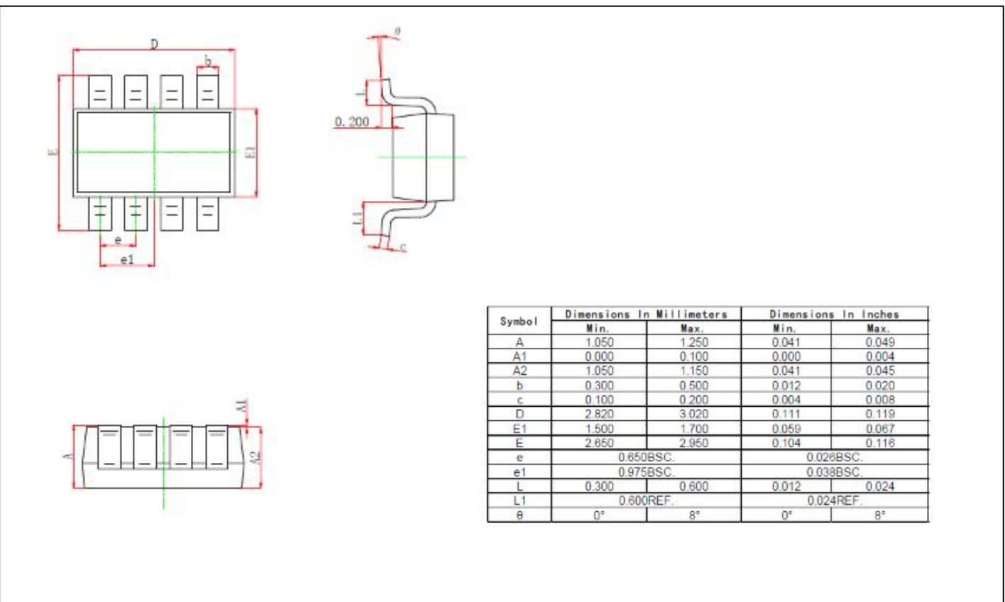
DIMENSIONS, SOT23-8L
