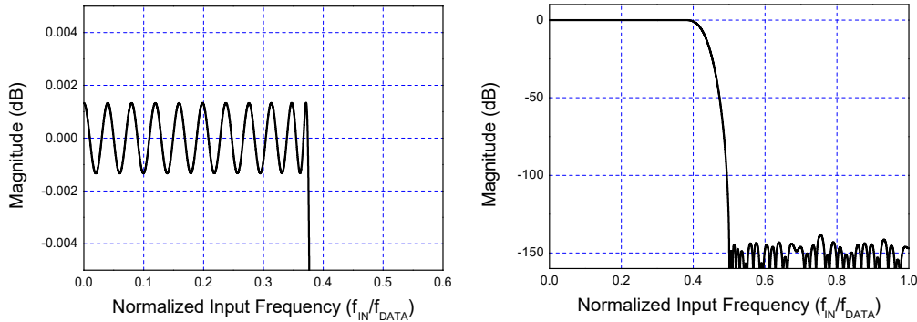
图 25 a) FIR 通带频率响应 b) FIR 过渡带频率响应
