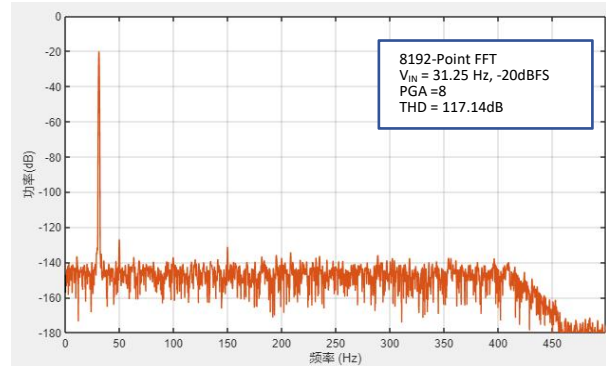
图 17 谐波 vs. 频率 @ PGA=8, 小信号输入
