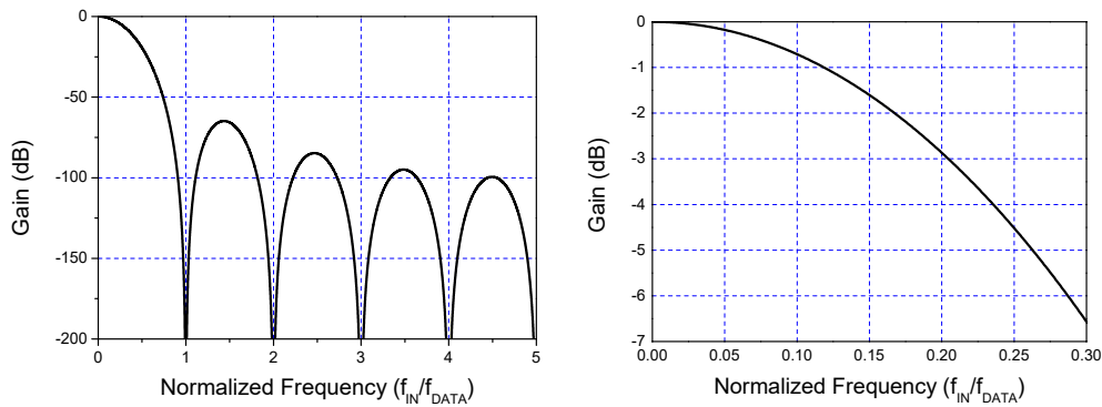
图 24 a) Sinc 滤波器频率响应 b) Sinc 滤波器滚降
