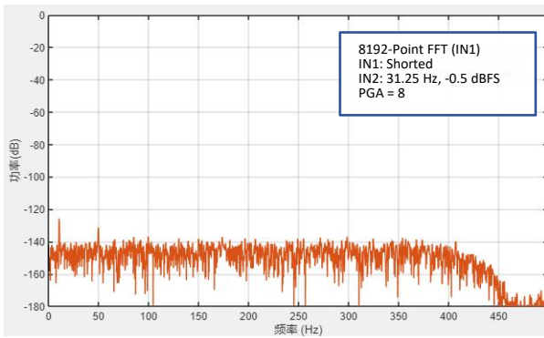
图 18 串扰频谱
