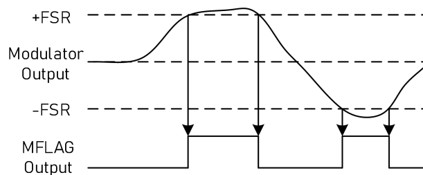
图 21 调制器过阈值监测原理
