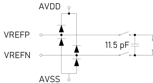
图 22 参考电压输入电路
