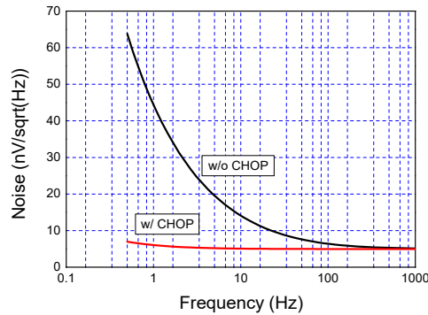
图 20 斩波开启/关断下的 PGA 噪声水平
