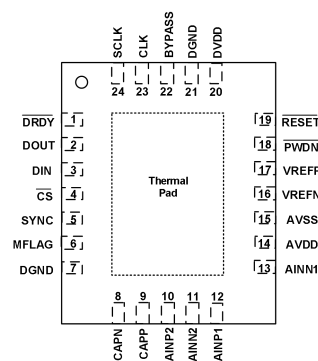
图 1 管脚定义
