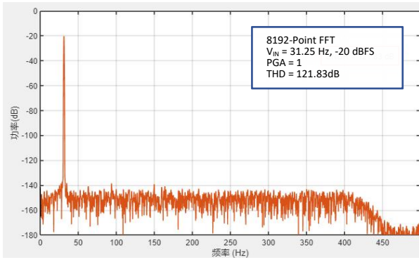
图 16 谐波 vs. 频率 @ PGA=1, 小信号输入
