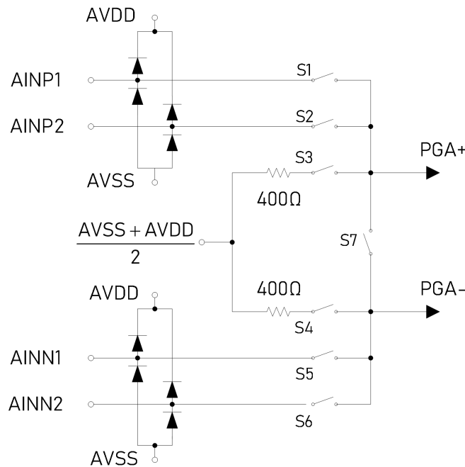
图 19 模拟输入多路复用器
