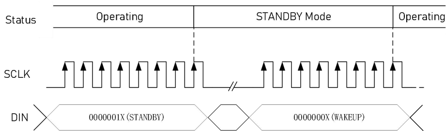
图 33 STANDBY 和 WAKEUP 指令时序
