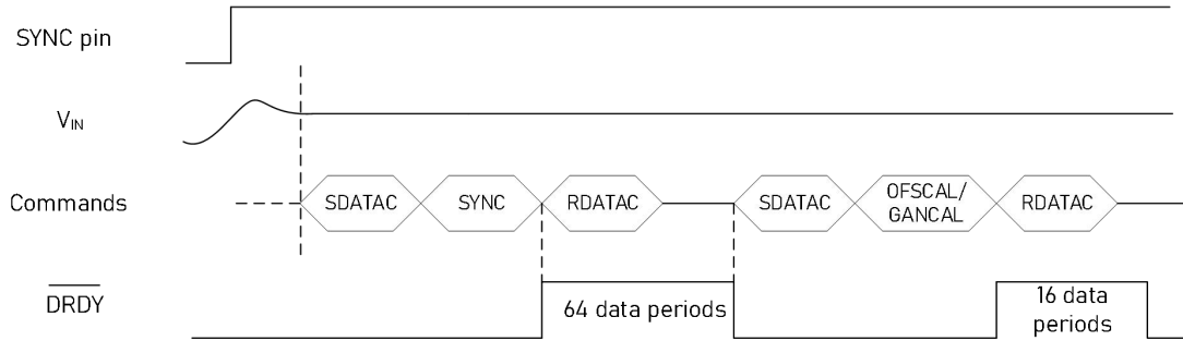
图 32 校正时序
