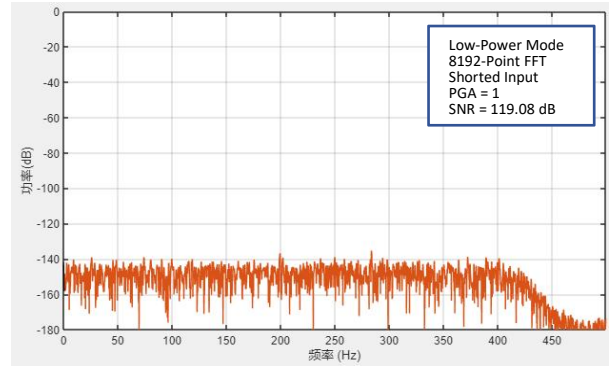
图 5 噪声 vs. 频率 @ PGA=1, 斩波模式 (低功耗模式)
