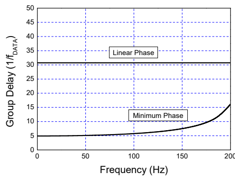
图 26 FIR 群延迟 ( f_{\text{DATA}} = 500\text{Hz} )
