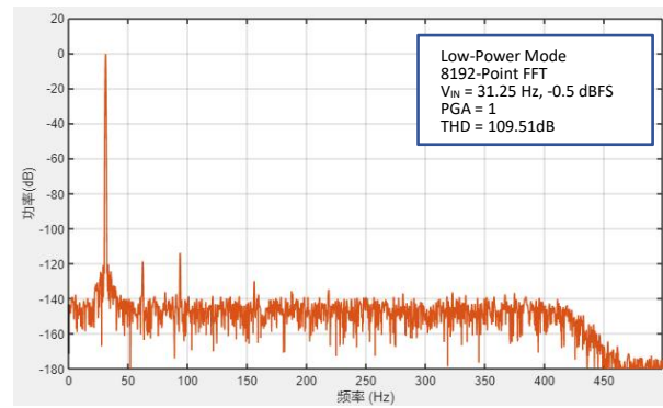
图 13 谐波 vs. 频率 @ PGA=1 (低功耗模式)
