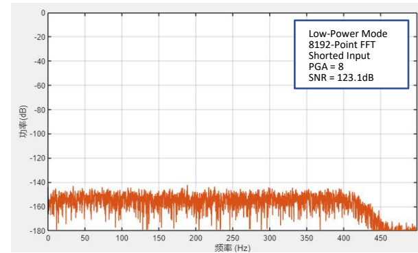
图 7 噪声 vs. 频率 @ PGA=8, 斩波模式 (低功耗模式)
