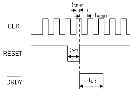
图 28 复位时序
