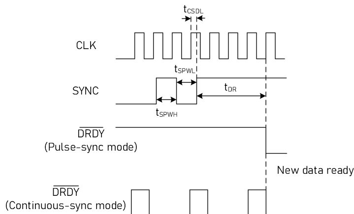
图 27 单脉冲触发的同步时序
