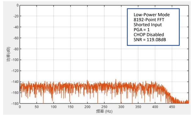
图 9 噪声 vs. 频率 @ PGA=1, 斩波模式关闭 (低功耗模式)
