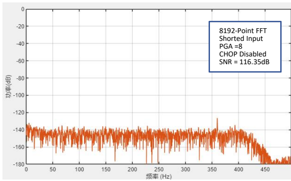
图 10 噪声 vs. 频率 @ PGA=8, 斩波模式关闭
