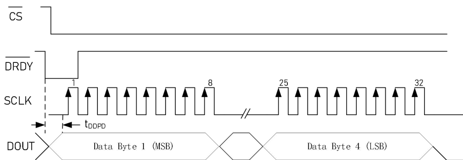
图 30 连续数据采集时序
