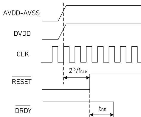
图 29 上电时序
