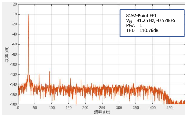
图 12 谐波 vs. 频率 @ PGA=1
