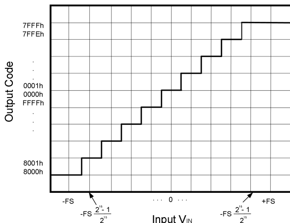
图 18 输出码转换曲线
