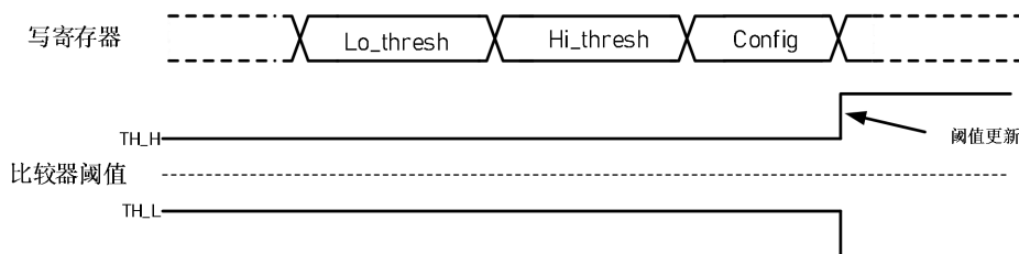
图 12 阈值寄存器写入时序
