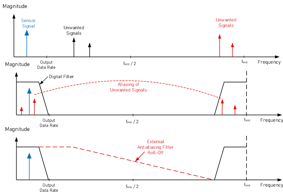
图 21 混叠效应示意图
