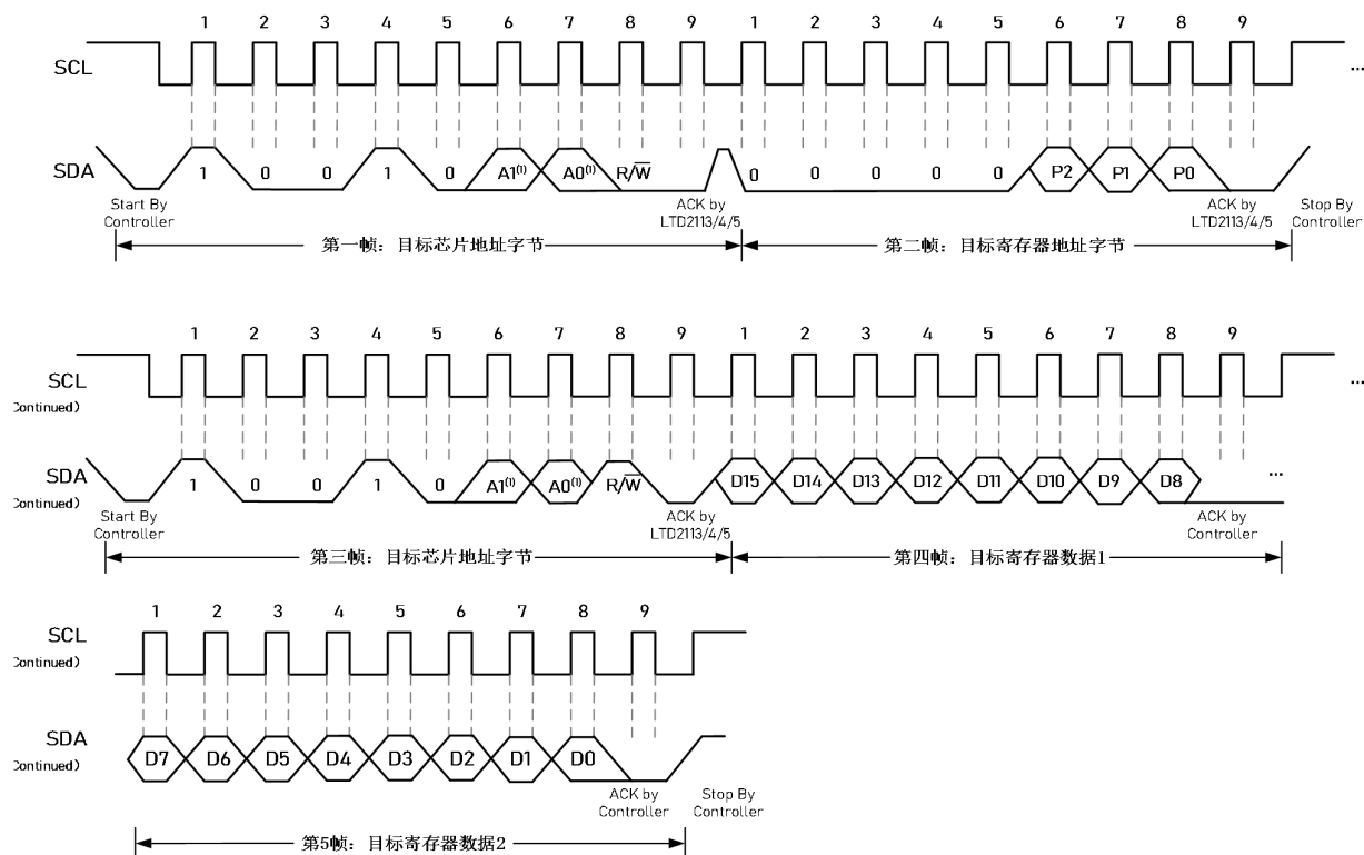
图 15 LTD211X 读时序
