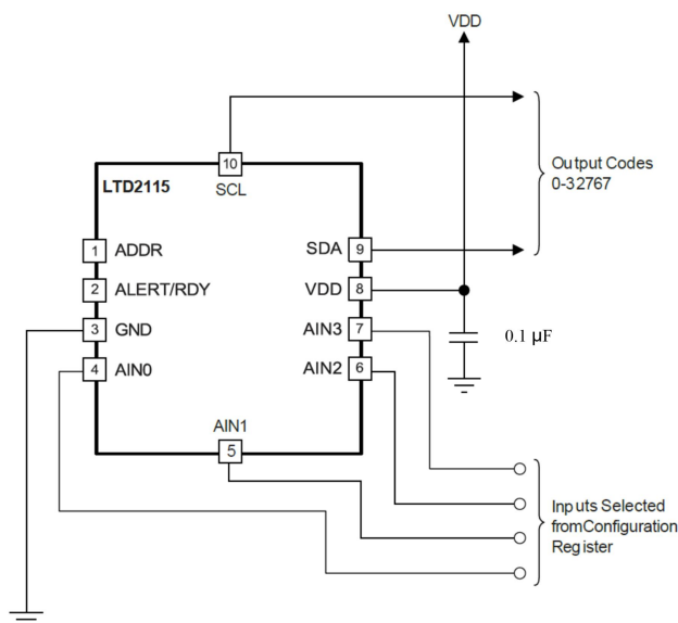
图 20 单端输入测量示例
