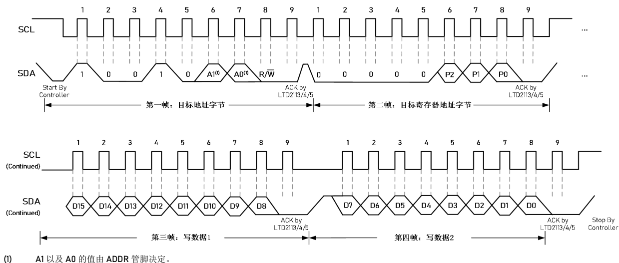
图 16 LTD211X 写时序
