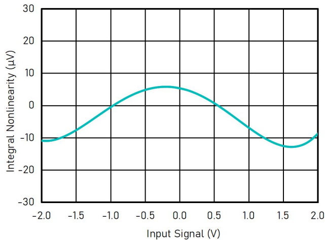
图5 INL 与输入信号的关系
