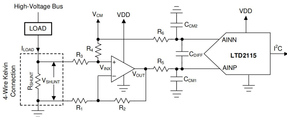
图 24 低侧电流分流监测电路图
