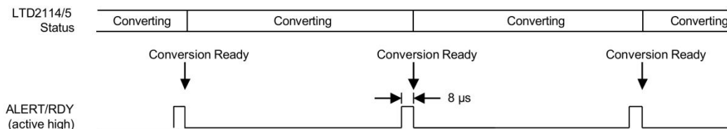
图 14 连续转换模式下的转换就绪脉冲
