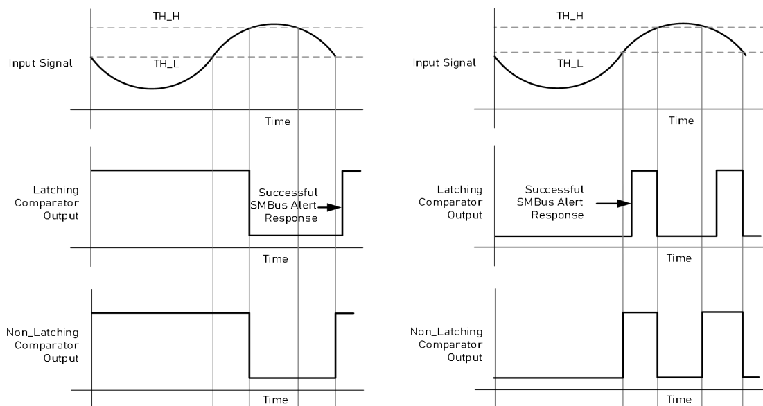
图 13 ALERT 引脚时序图(传统与窗口比较器模式)
