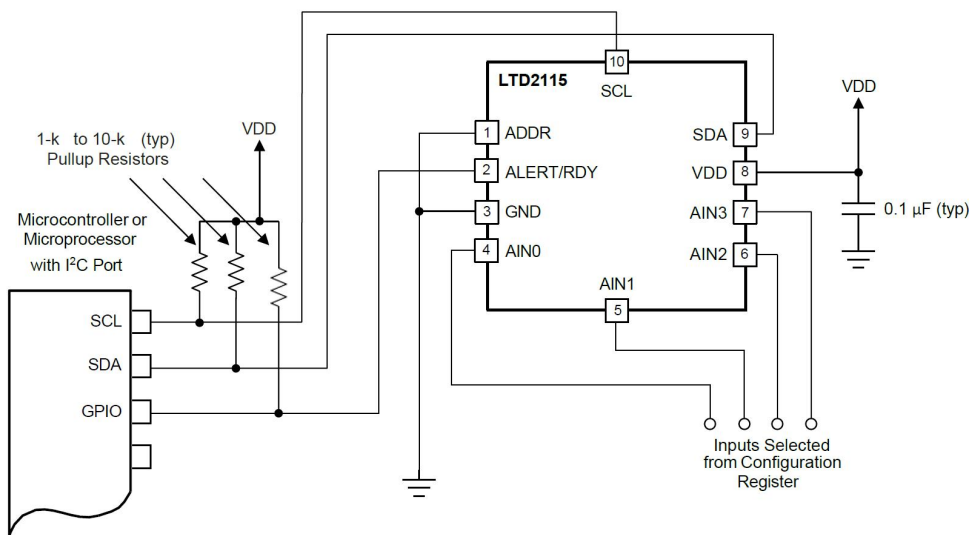
图 19 LTD2115 典型连接示例
