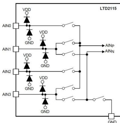
图 9 模拟输入电路示意图
