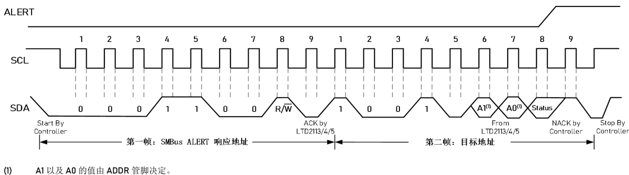
图 17 Alert 响应时序
