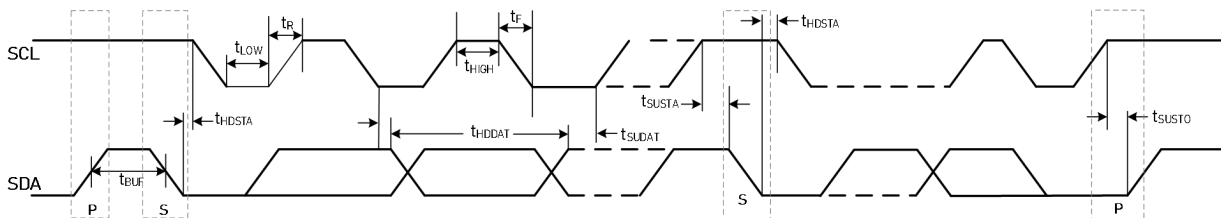
图 2 I²C 接口时序图
